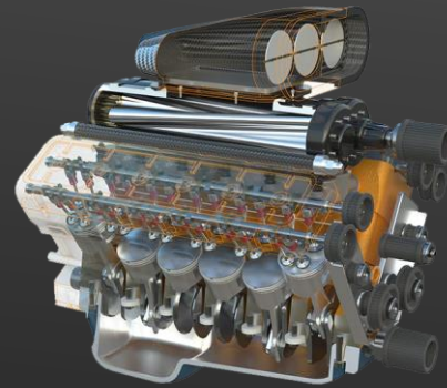
V8 Motor (3D Konstruktion)
